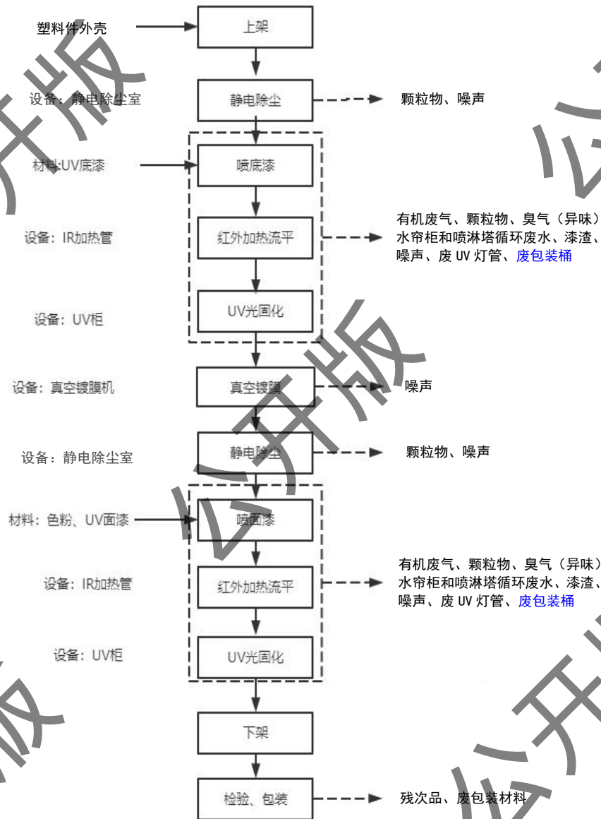
图 2-4 喷涂生产工艺流程图
